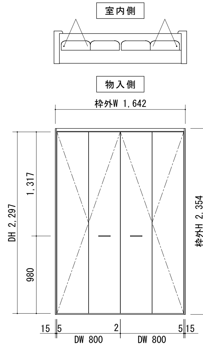
正面図
